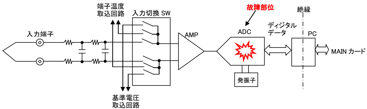
入力部ブロック図
