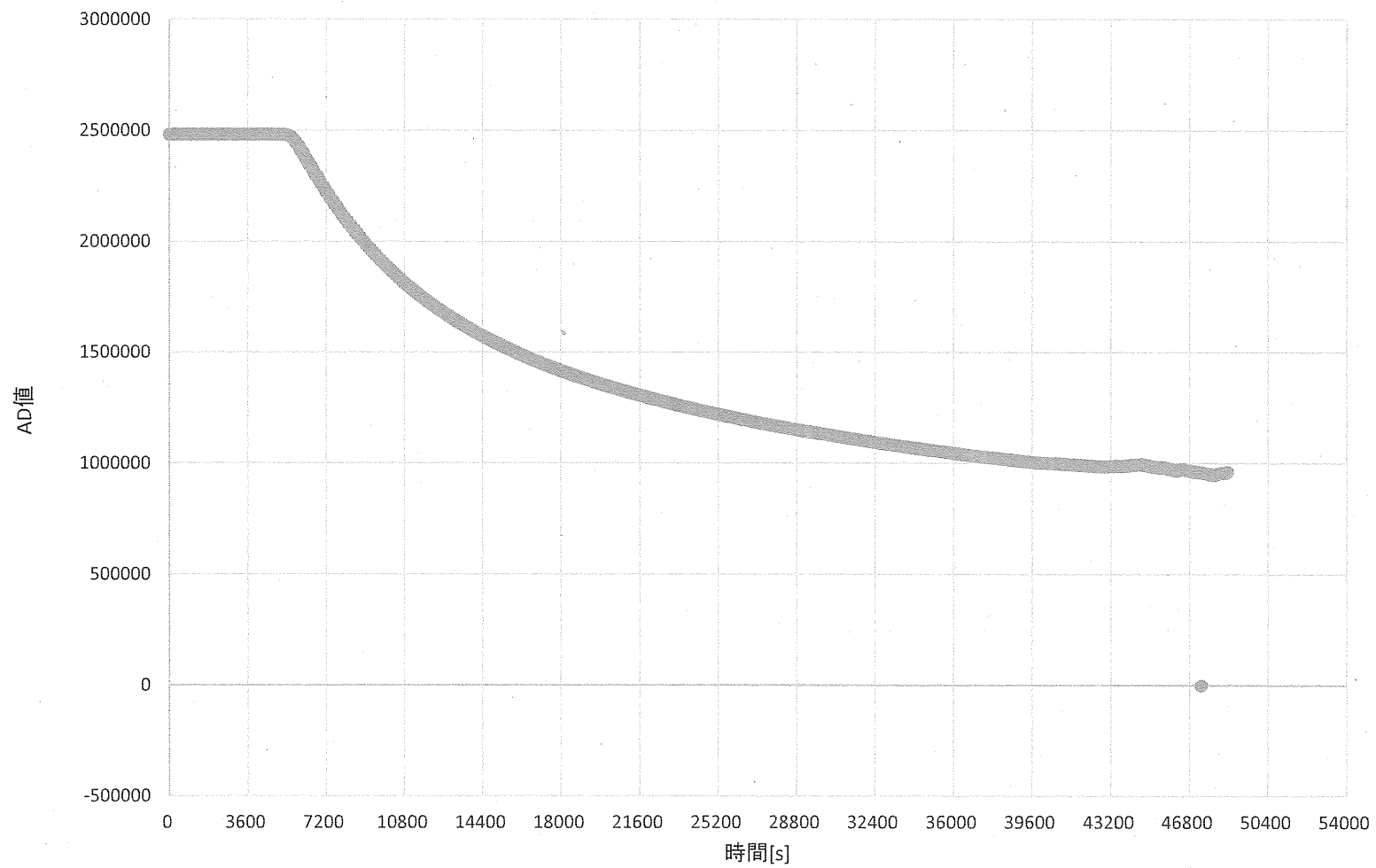
図 AIN4-AIN5間のAD値図
