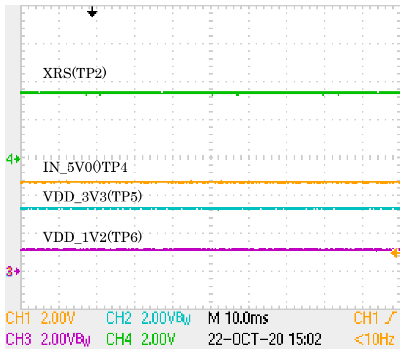
CCS-デバック MODE 開始直後の波形
